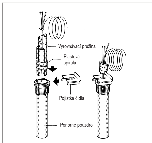
Obr. 10 – Schématické znázornění
