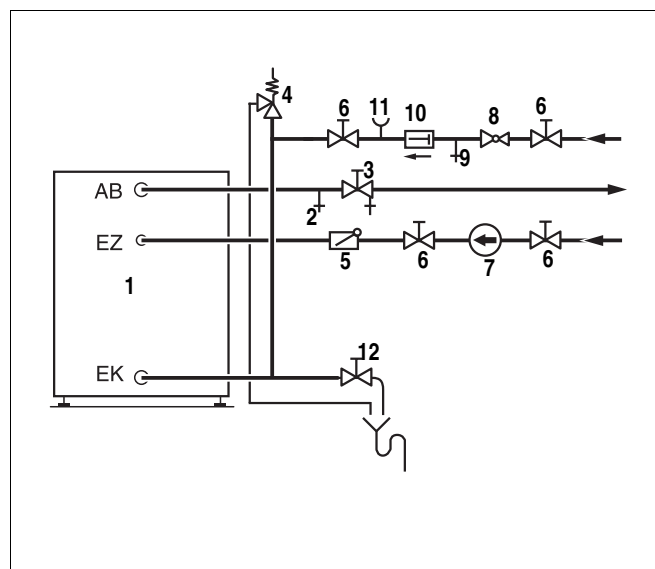
Obr. 3 Instalace a vybavení potrubí užitkové vody
