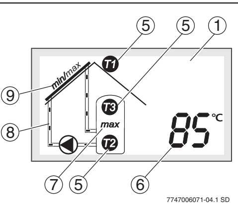
Rys. 9 Stacja solarna
