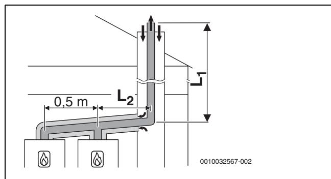
Obz. 29 Kaskáda se 2 zařízeními: Pevná spalinová cesta podle C 93x v šachtě a koaxiální systém odvodu spalin v místě instalace
