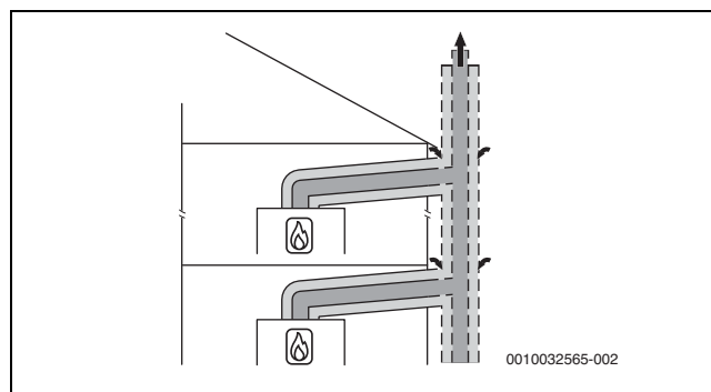
Obr. 24 Zapojení několika tepelných zdrojů do jednoho spalínového zařízení podle C_{(12)3x} pomocí koaxiálního systému odvodu spalin v místě instalace
