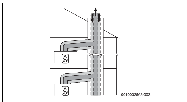
Obr. 23 Zapojení několika tepelných zdrojů do jednoho spalínového zařízení podle C_{(10)3x} pomocí koaxiálního systému odvodu spalin v místě instalace
