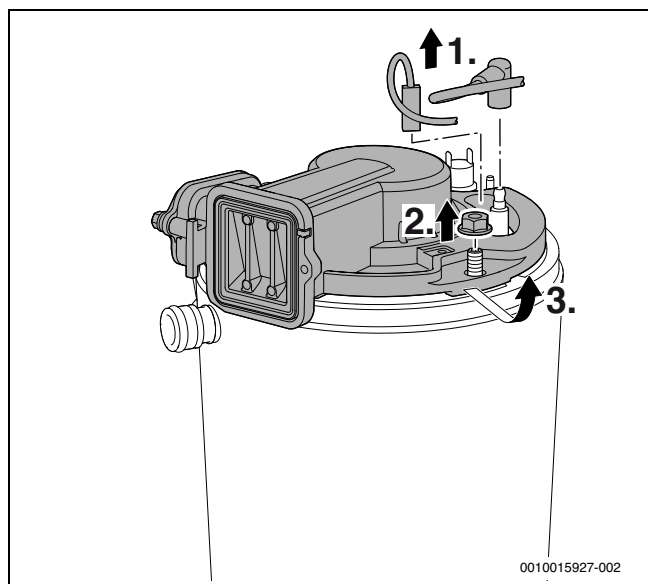
Obr. 53 Uvolnění krytu hořáku
