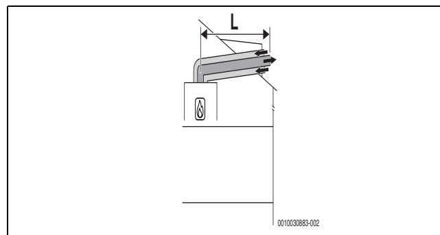
Obr. 6 Horizontální koaxiální systém odvodu spalin podle C 13x přes střechem
