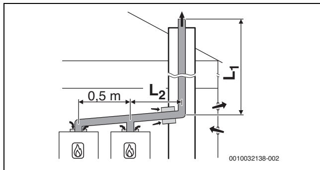
Obr. 28 Kaskáda se 2 zařízeními: Pevné vedení odtahu spalín v šachtě podle B 53p s přívodem vzduchu závislým na vzduchu z prostoru na zařízení
