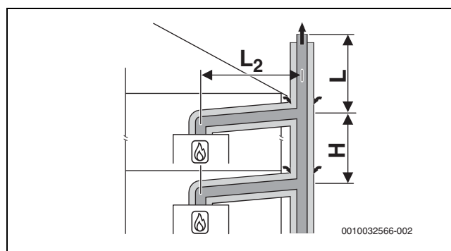
Obr. 25 Zapojení několika tepelných zdrojů do jednoho spalínového zařízení podle C_{(13)3x} pomocí koaxiálního systému odvodu spalin po venkovní stěně a v místě instalace
