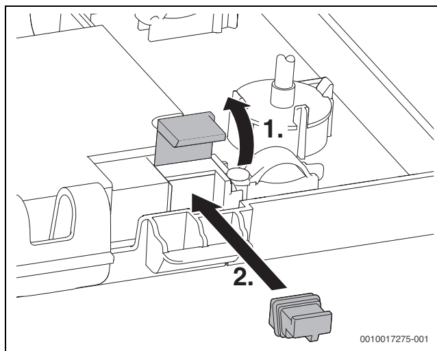
Obr. 78 Zasunutí kódovacího konektoru
