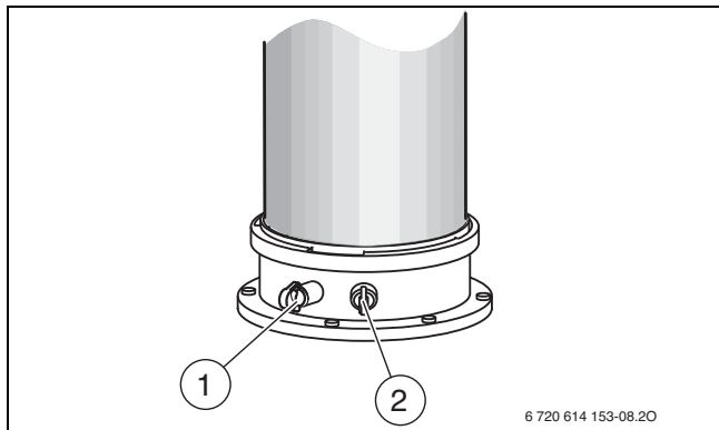
Obr. 50 Měřicí hrdlo spalín a měřicí hrdlo spalovacího vzduchu
