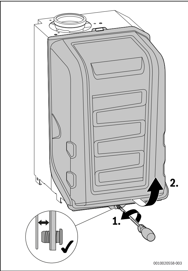
Obr. 57 Sejmutí krytu hořáku
