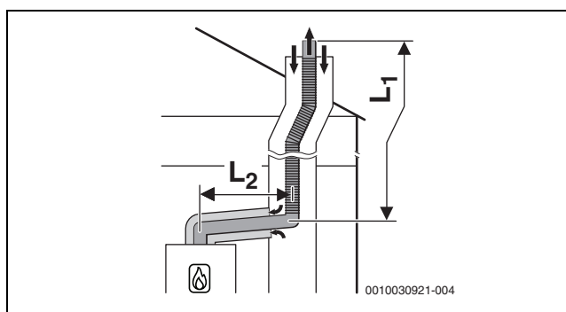
Obr. 24 Flexibilní spalínová cesta podle C 93x v šachtě a koaxiální systém odvodu spalín v místě instalace
