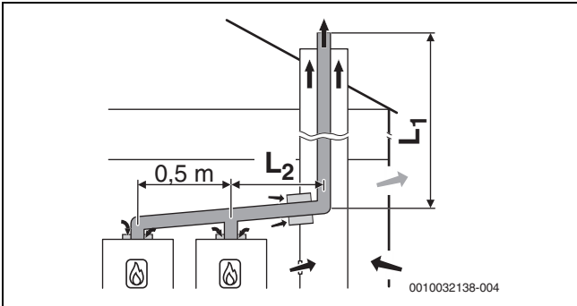
Obr. 27 Kaskáda se 2 zařízeními: Pevné vedení odtahu spalin v šachtě podle B 53p s přívodem vzduchu závislým na vzduchu z prostoru a jednotěnným
