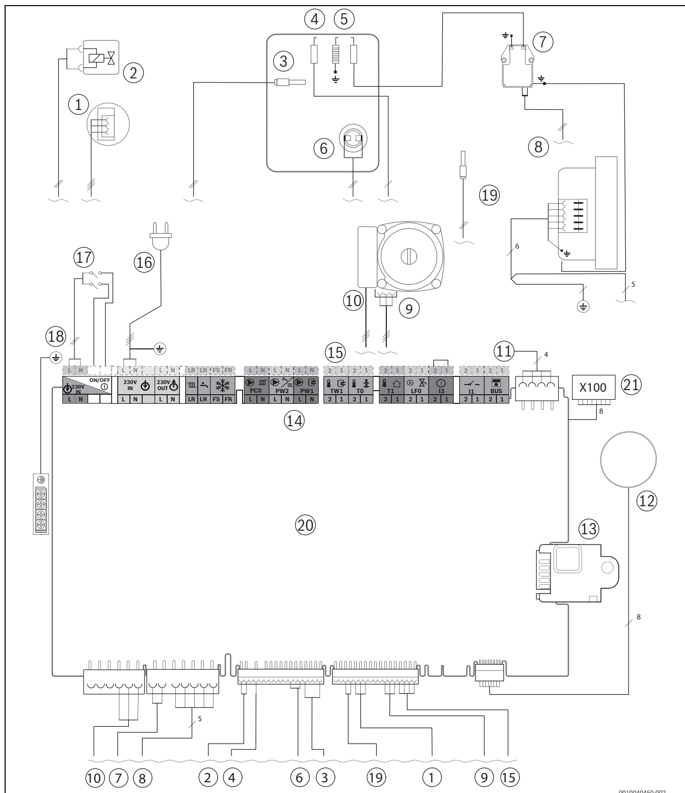
Obr. 80 Elektrické kabelové propojení
