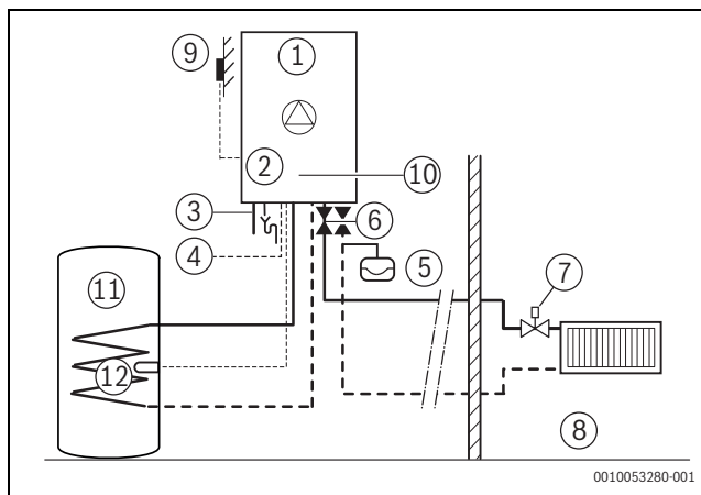
Obr. 37 Příklad použití s regulací řízenou podle venkovní teploty a zásobníkem teplé vody
