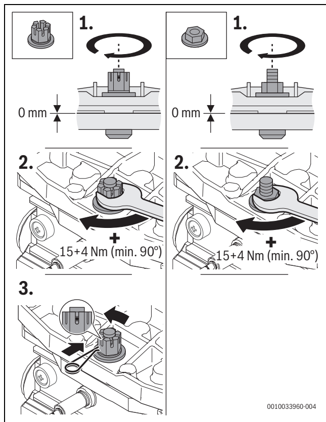
Obr. 65 Utažení matice na krytu hořáku
