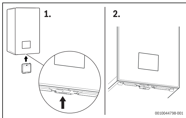
Obr. 49 Poloha konektoru pro přídavný modul
