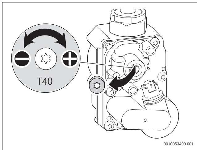
Obr. 60 Nastavení obsahu CO 2 nebo O 2
