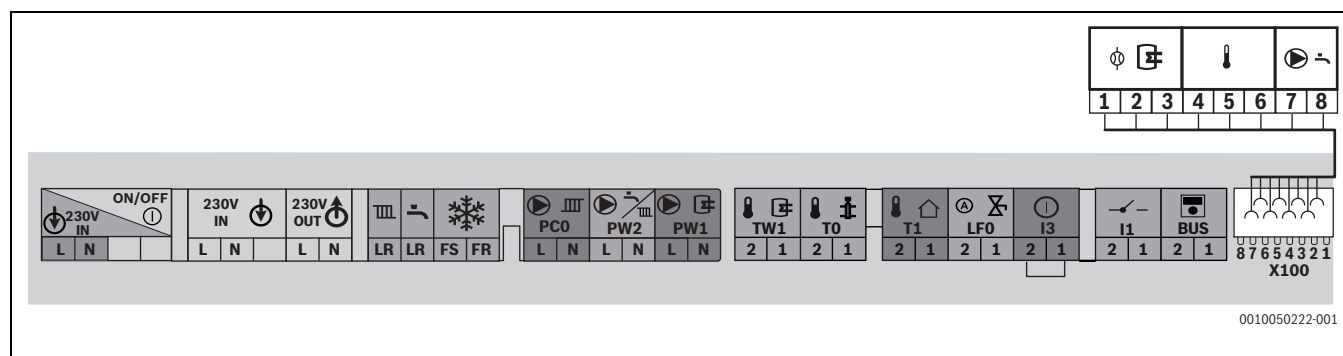
Obr. 45 Svorkovnice pro externí příslušenství
