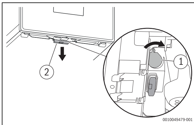
Obr. 50 Demontáž Connect-Key
