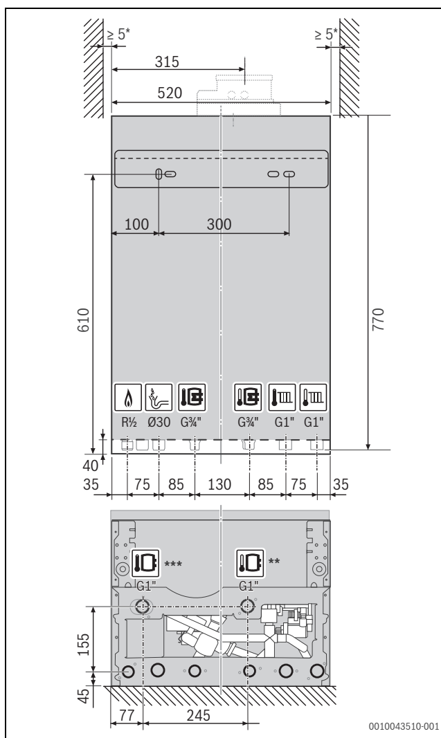
Obr. 4 Čelní pohled GB192i.2 15-35 kW (T40S)(mm)
