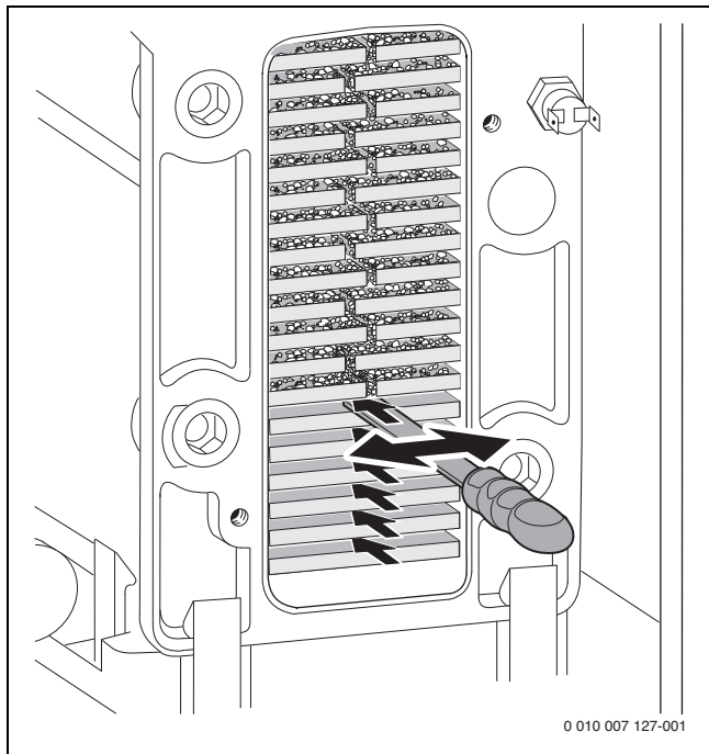
Obr. 69 Čistící nůž
