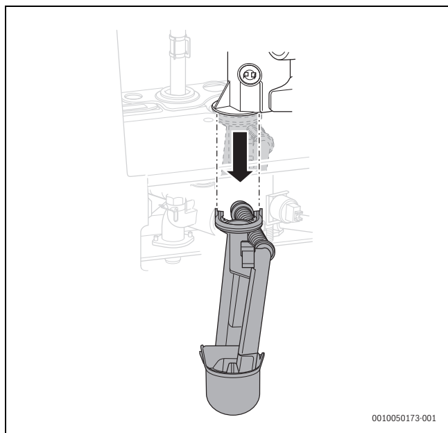
Obr. 73 Sifon kondenzátu
