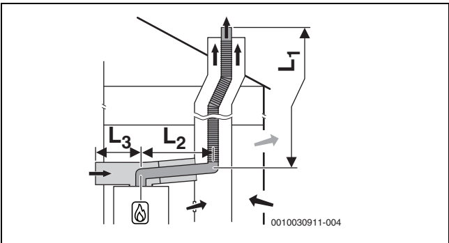
Obr. 19 Flexibilní spalínová cesta podle C 53x v šachtě a systém odvodu spalín se samostatným přívodem vzduchu a koaxiálním vedením odtahu spalín v místě instalace
