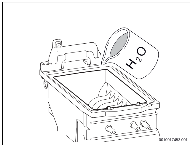
Obr. 71 Výplach tepelného bloku
