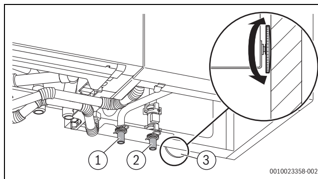
Obr. 40 Přípojky vody zásobníku 40 l
