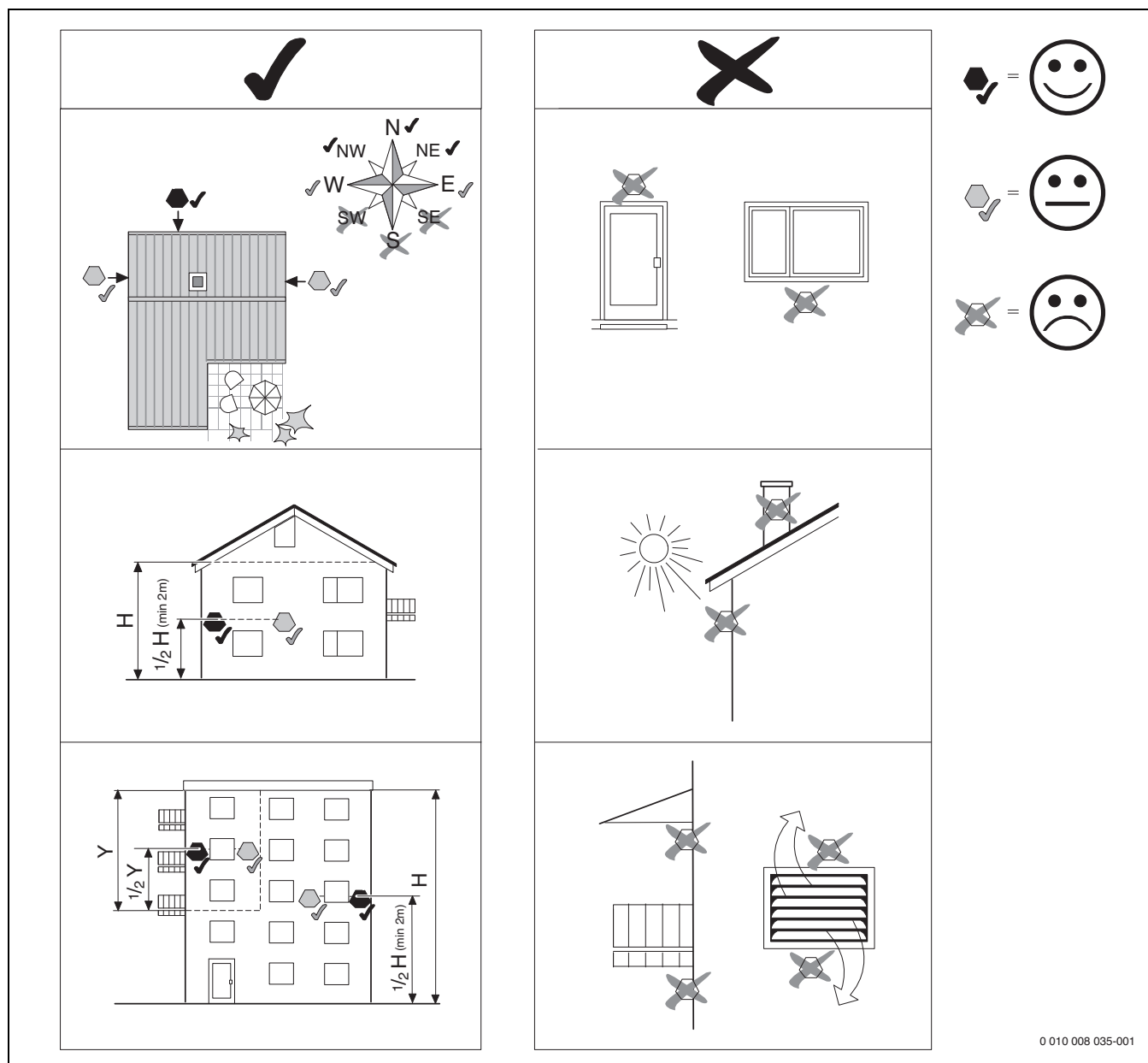
Obr. 35 Místo instalace čidla venkovní teploty (při regulaci řízené podle venkovní teploty s nebo bez korekce podle teploty prostoru)
