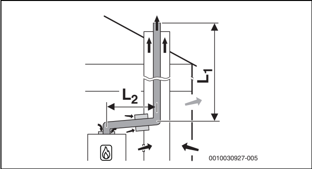
Obr. 25 Pevné vedení odtahu spalin v šachtě podle B 53p s přívodem vzduchu závislým na vzduchu z prostoru a jednotěnným vedením odtahu spalin v místě instalace; vzduchová mřížka v šachtě
