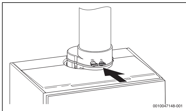
Obr. 59 Měřicí bod spalín
