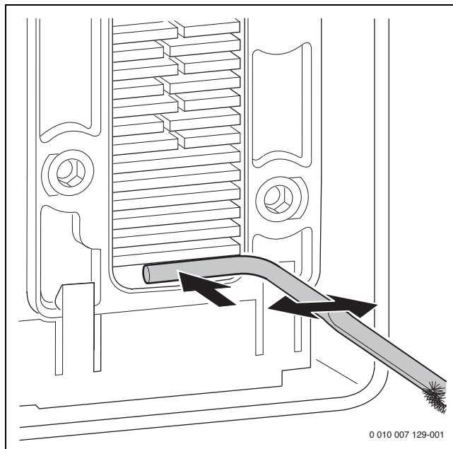
Obr. 72 Čištění vany na kondenzát
