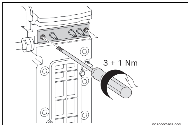
Obr. 61 Montáž sady elektrod
