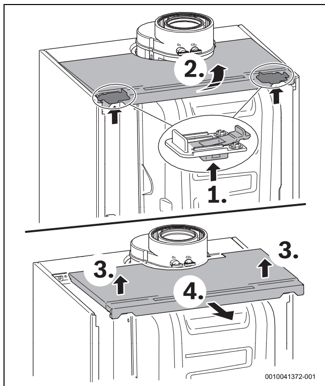
Obr. 52 (De)montáž opláštění
