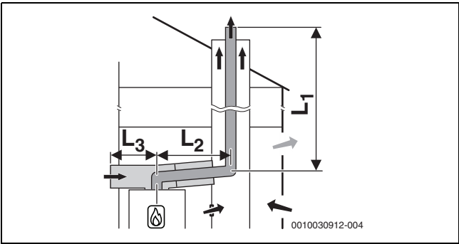
Obr. 18 Pevná spalínová cesta podle C 53x v šachtě a systém odvodu spalín se samostatným přívodem vzduchu a koaxiálním vedením odtahu spalín v místě instalace
