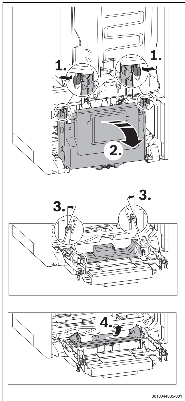
Obr. 43 Otevření řídicí jednotky
