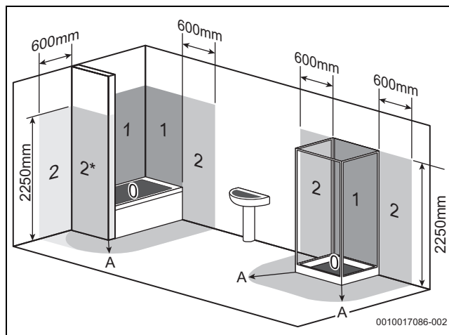
Obr. 29 Ochranné úseky (příklad)
