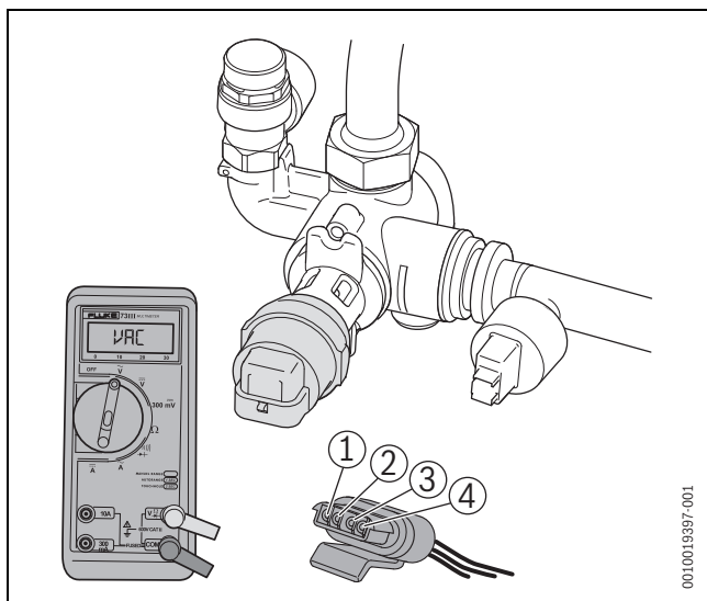
Obr. 77 3-Wege-Ventil
