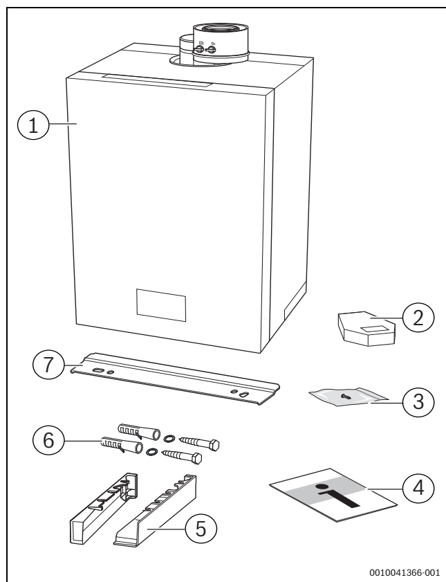
Obr. 1 Rozsah dodávky
