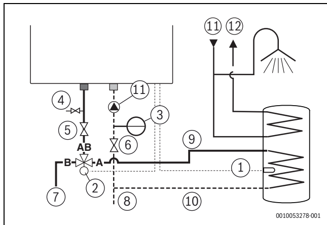
Obr. 38 Montáž externího 3cestného ventilu (230 V)
