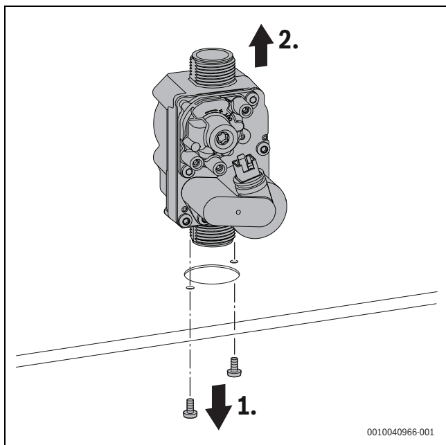
Obr. 76 Demontáž plynového ventilu
