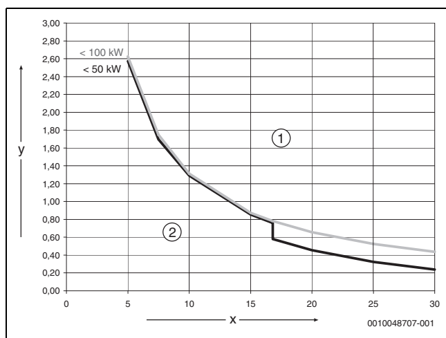
Obr. 30 Zdroj tepla &lt; 50 kW &lt; 100 kW
