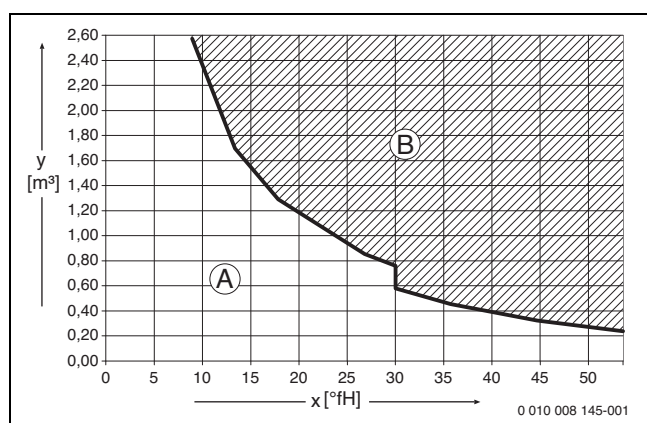
Obr. 32 Požadavky na plnicí a doplňovací vodu v °fH u zařízení < 50 kW
