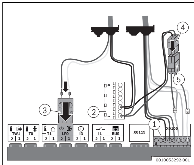
Obr. 48 Připojení zásobníku teplé vody
