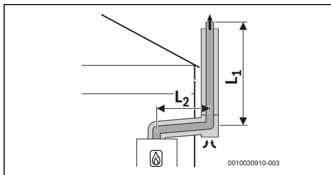
Obr. 22 Koaxiální systém odvodu spalin podle C 53x na venkovní stěně
