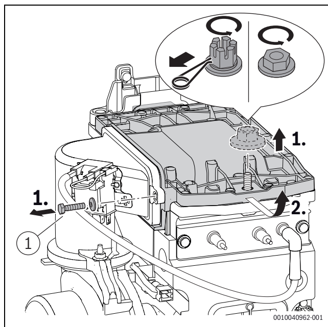
Obr. 63 Odmontování krytu hořáku
