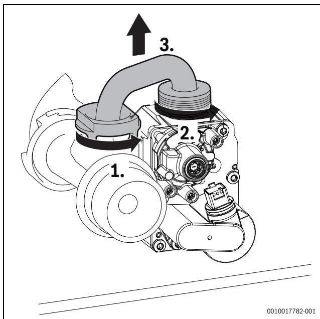
Obr. 74 Odmontování plynového potrubí
