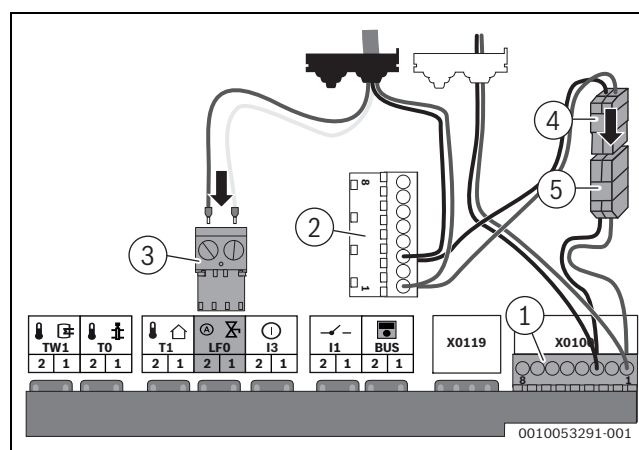
Obr. 47 Připojení automatického plnicího ventilu pro zařízení GBH192i.2-1
