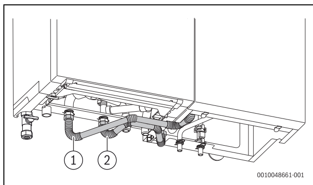
Obr. 39 Propojení zásobníku teplé vody a zařízení
