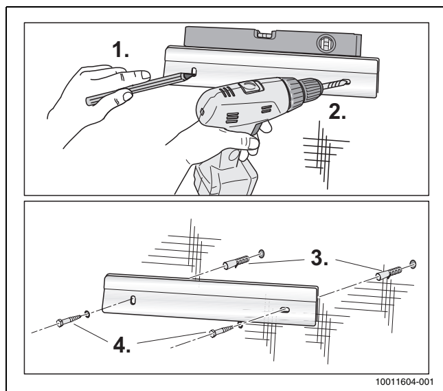
Obr. 33 Montáž závěsné lišty
