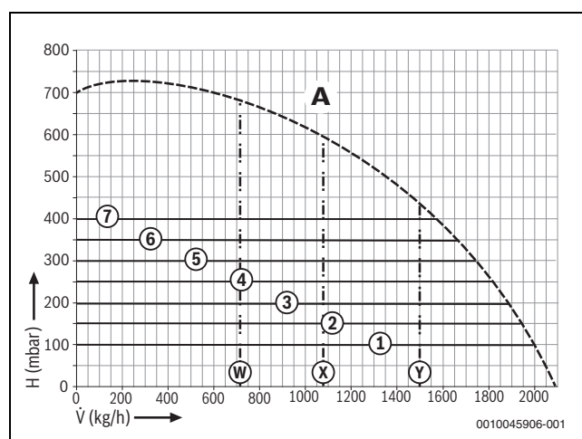
Obr. 78 GB192i.2-15(W) HGB192i.2-25(W) HGB192i.2-30 T40SW H a GB192i.2-35(W) H: Pole charakteristik čerpadla a charakteristiky čerpadla
