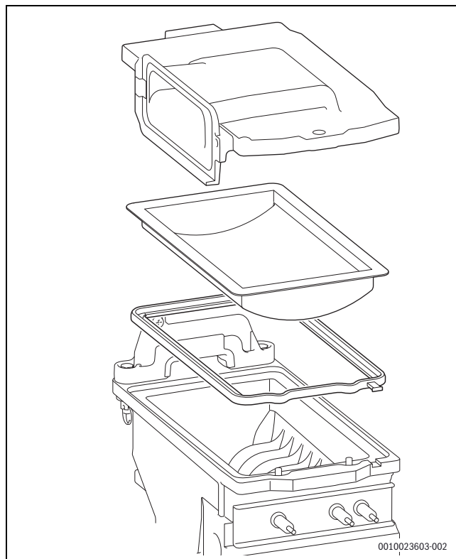
Obr. 64 Hořák
