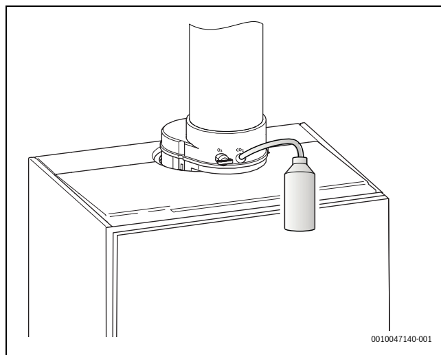
Obr. 41 Naplnění sifonu kondenzátu vodou
