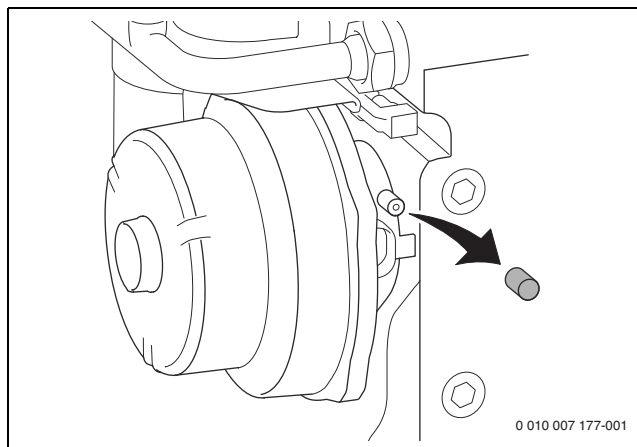
Obr. 68 Měřicí hrdlo na směšovacím zařízení
