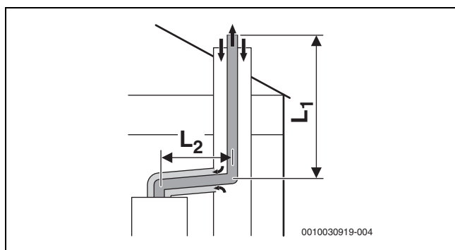
Obr. 23 Pevná spalínová cesta podle C 93x v šachtě a koaxiální propojovací potrubí v místě instalace
