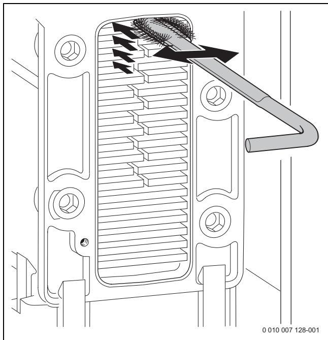
Obr. 70 Čištění tepelného bloku kartáčem
