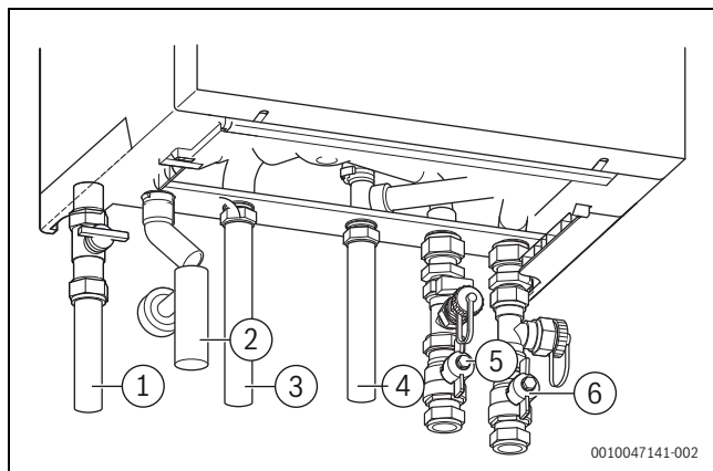
Obr. 36 GB192i.2 Přípojky vody a plynu (příslušenství)
