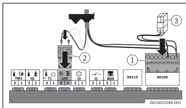
Obr. 46 Připojení automatického plnicího ventilu pro systémová zařízení / Pouze nástěnné kotle
