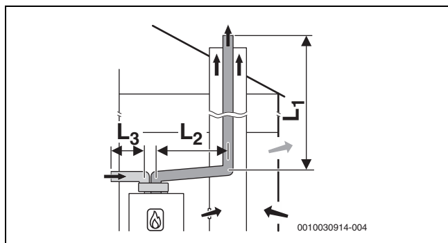
Obr. 20 Pevná spalinová cesta podle C 53 v šachtě a oddělená jednotěnná vedení vstupu vzduchu a odtahu spalin v místě instalace
