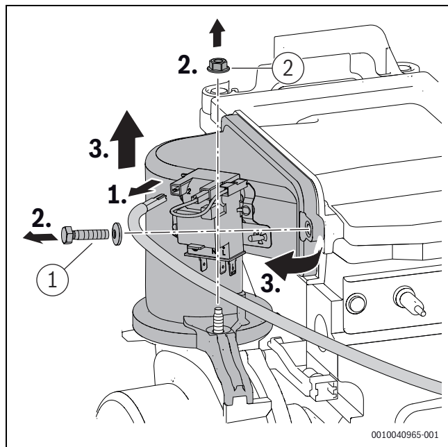
Obr. 66 Vymontování směšovacího zařízení
