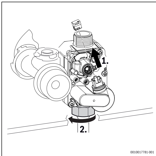
Obr. 75 Odpojení konektoru a povelení převlečné matice
