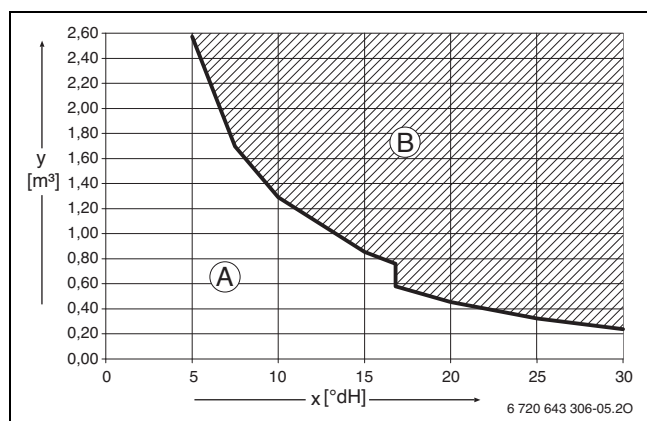
Obr. 31 Požadavky na plnicí a doplňovací vodu v °dH u zařízení < 50 kW
