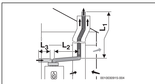
Obr. 21 Flexibilní spalinová cesta podle C 53 v šachtě a oddělená jednotěnná vedení vstupu vzduchu a odtahu spalin v místě instalace
