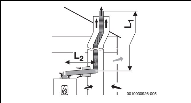
Obr. 26 Flexibilní vedení odtahu spalin v šachtě podle B 53p s přívodem vzduchu závislým na vzduchu z prostoru a jednotěnným vedením odtahu spalin; vzduchová mřížka v šachtě
