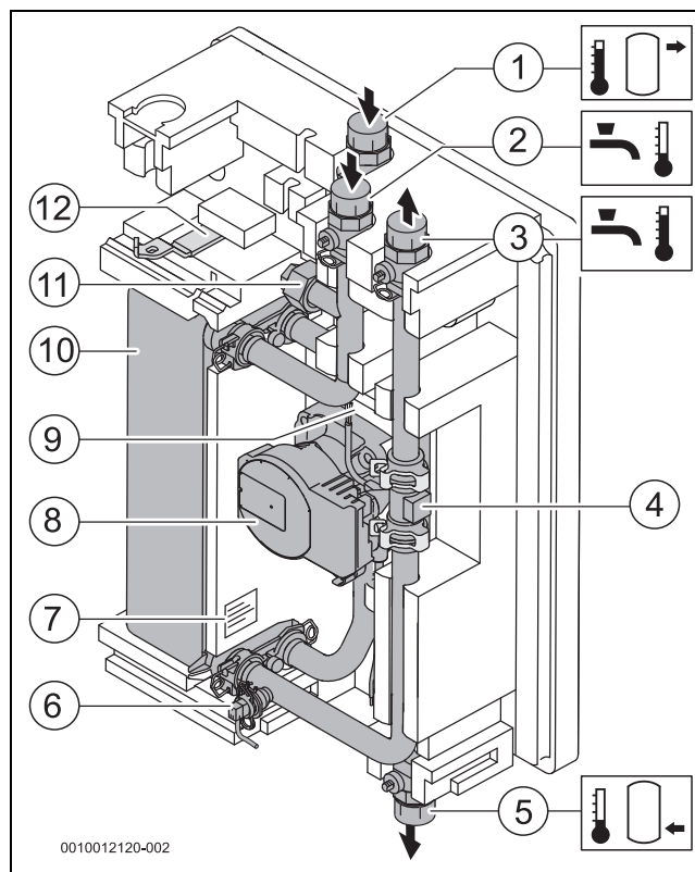
Obr. 2 Stanice pro přípravu teplé vody bez přední tepelné izolace, bez modulu
