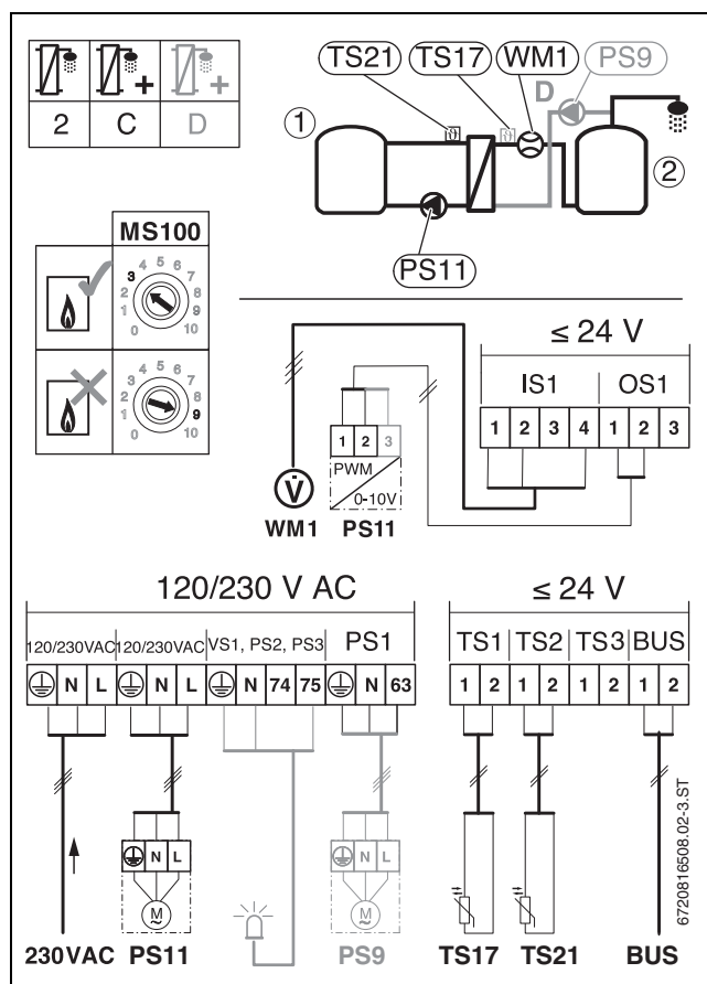
Obr. 33 Připojovací svorky u předehřívací stanice pro přípravu teplé vody
