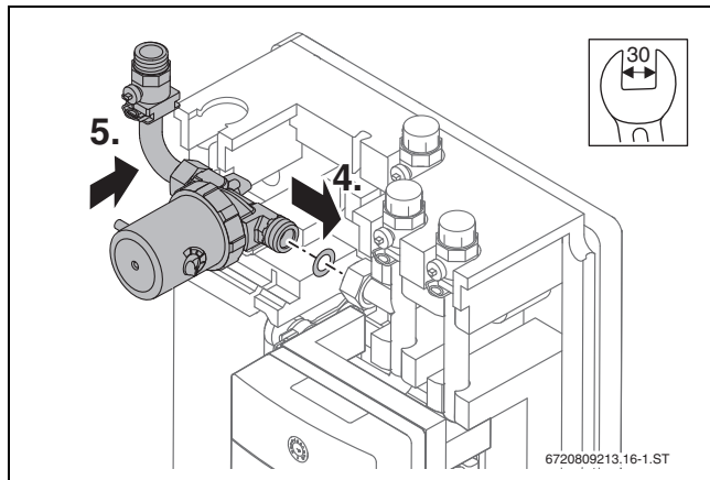
Obr. 23 Příprava montáže
