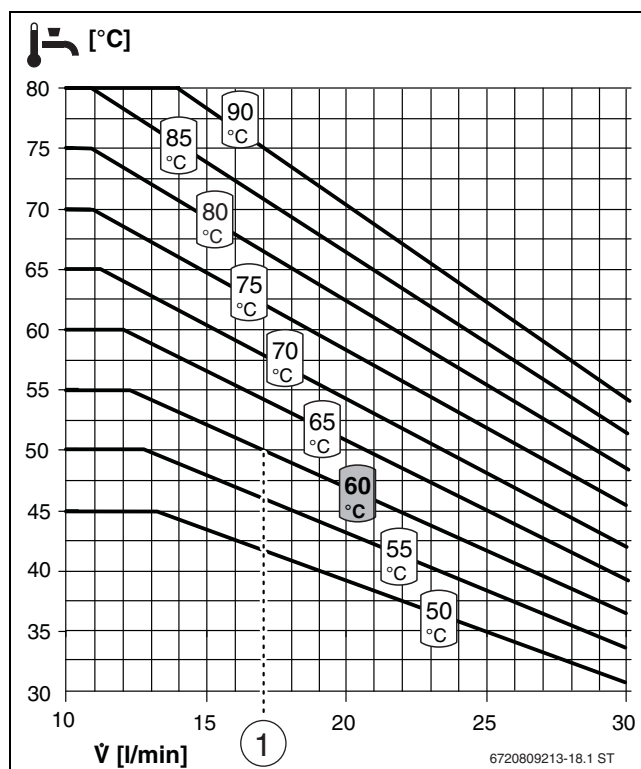
Obr. 38 Chování teploty FS/2
