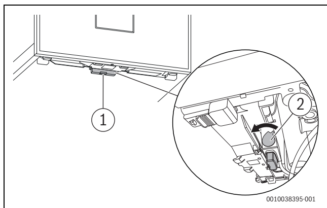
Obr. 5 Zajištění Key
