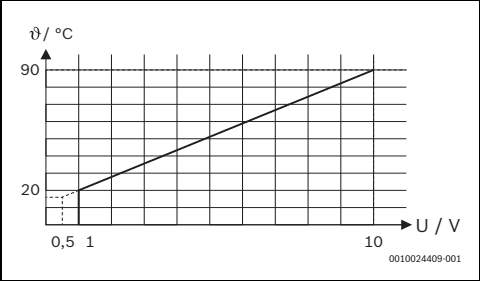
Afb. 2 Lineaire relatie tussen 0-10 V-signaal (U in V) en gevraagde aanvoertemperatuur (9 in °C)
