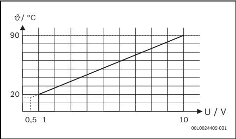
Obr. 2 Lineární závislost mezi signálem 0-10 V (U ve V) a požadovanou teplotou na výstupu (θ ve °C)
