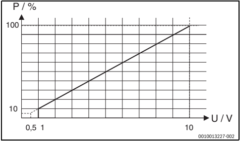
Obr. 1 Lineární závislost mezi signálem 0-10 V (U ve V) a požadovaným výkonem (P v %)
