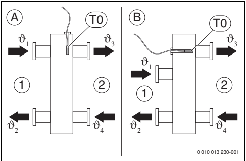
Fig. 3 Posizione sonda di temperatura mandata (T0)
